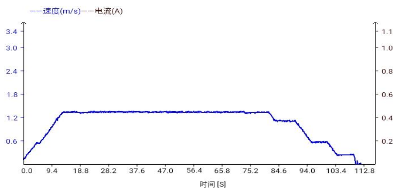
图 2. 提升系统 I. V 曲线图
