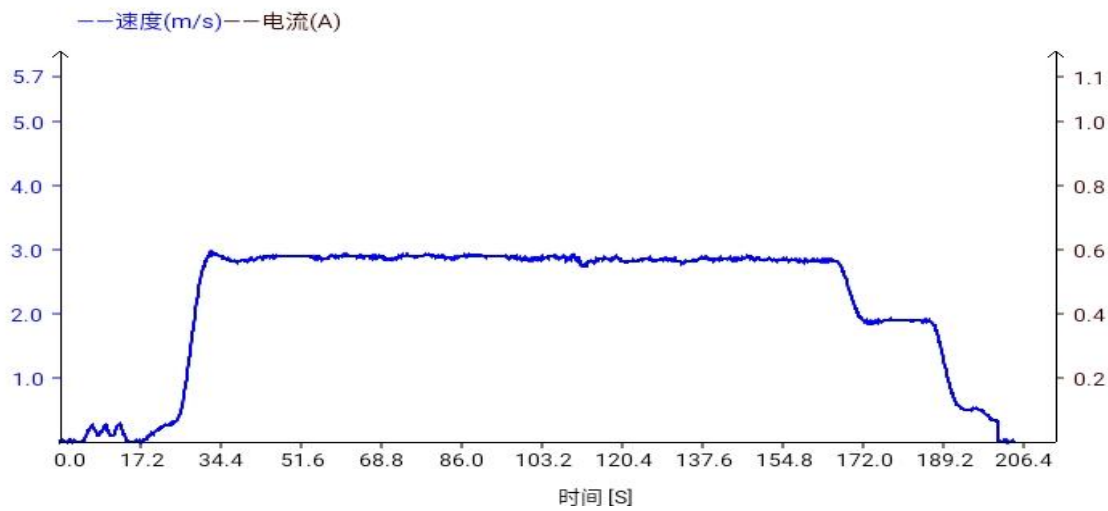
图 1 提升机 I、v 上提曲线图
