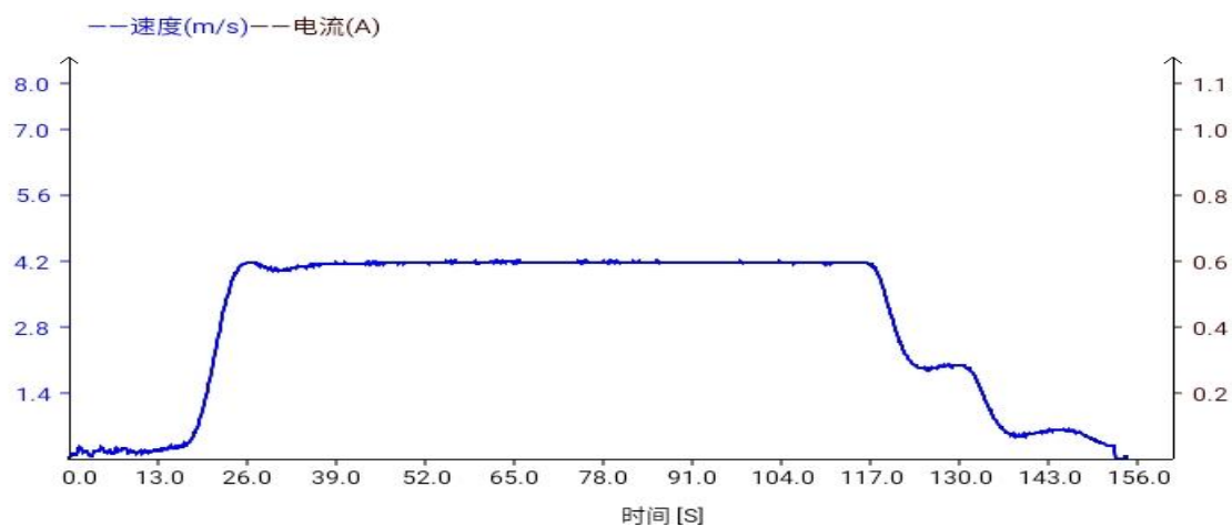
图 2 提升机 I、v 上提曲线图
