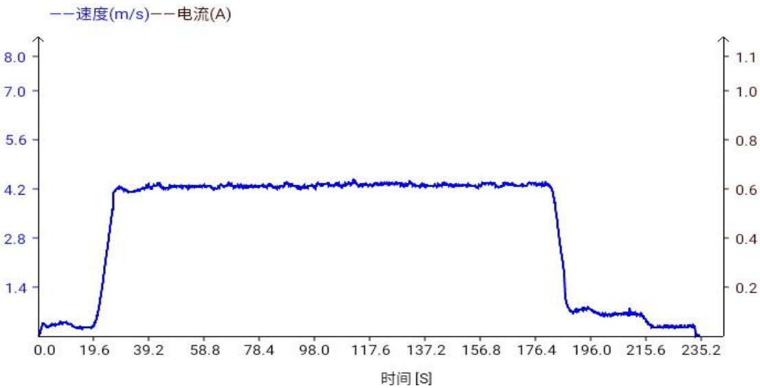
图 1. 提升系统 I. V 曲线图
