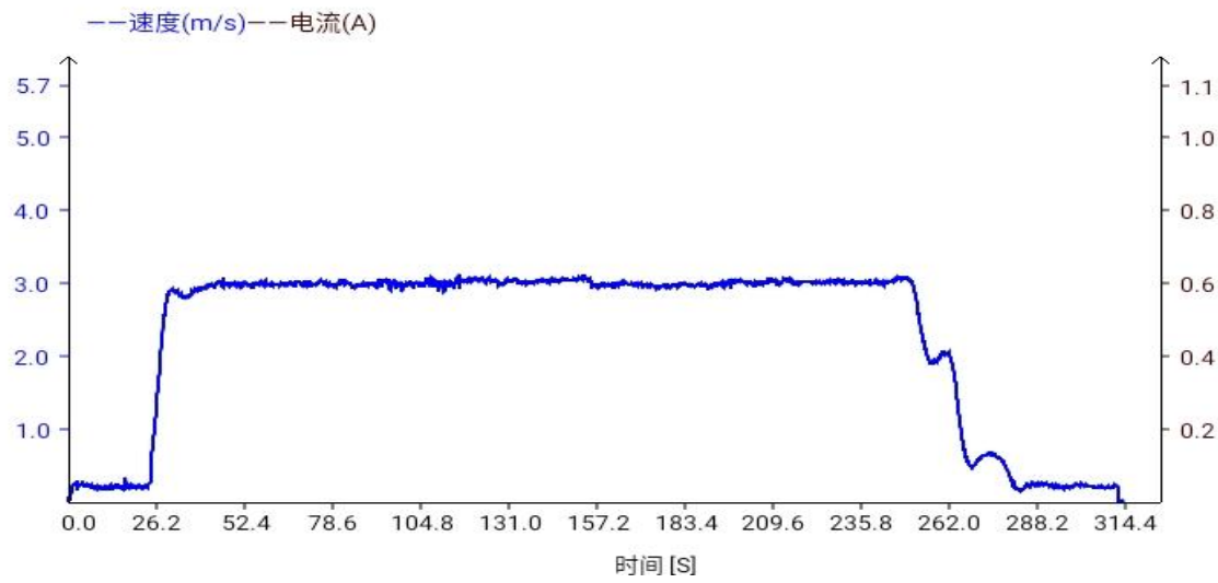
图 2. 提升系统 I. V 曲线图
