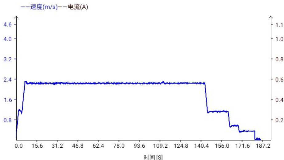
图 1 提升机 I、v 上提曲线图
